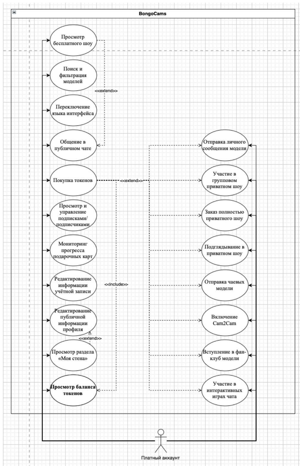
Рисунок 3 - UseCase диаграмма прецедентов для роли Платный аккаунт
